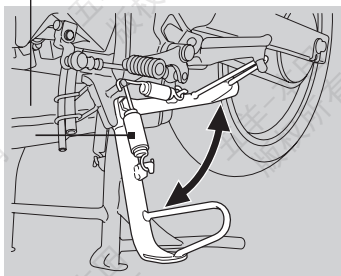
侧支架弹簧
