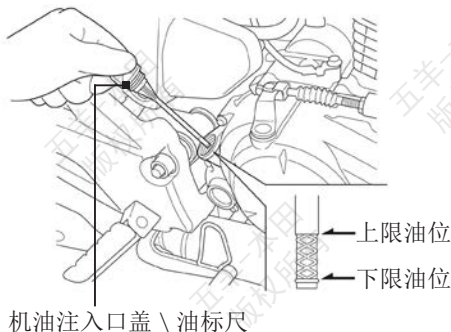
机油注入口盖 \ 油标尺
