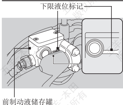
前制动液储存罐
