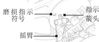
后制动鼓刹
