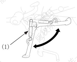
(1) 侧支架弹簧
