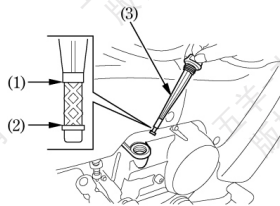
(1) 上限标位 (2) 下限标位 (3) 机油标尺
