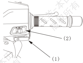
(1) 电起动开关 (2) 照明开关
