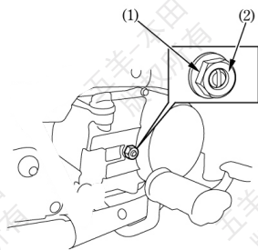
(1) 调节螺钉锁紧螺母 (2) 离合器调节螺钉
