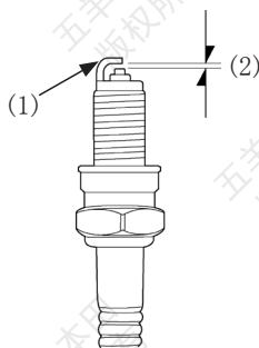
(1) 侧电极
