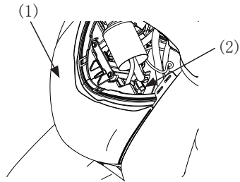
(1) 前照灯 (2) 调节螺杆
