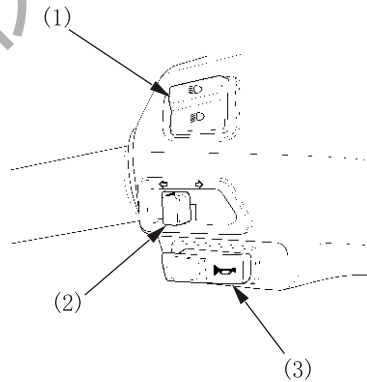
(1) 前照灯变光开关 (2) 转向信号开关 (3) 喇叭按钮
