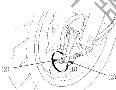
(2) 前制动调节螺母 (3) 制动臂连接销
