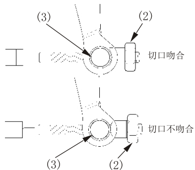
(A) 自由行程减少 (B) 自由行程增大
