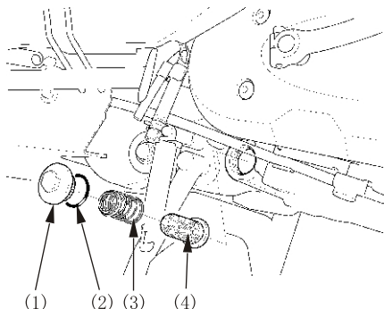
(1) 泄油管塞 (2) O型密封环 (3) 弹簧 (4) 机油滤网
