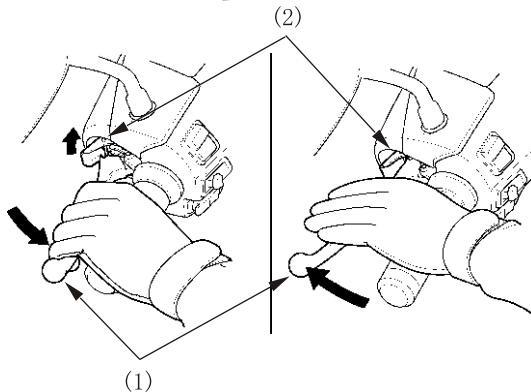
(1) 后制动手柄 (2) 后制动手柄止动板
