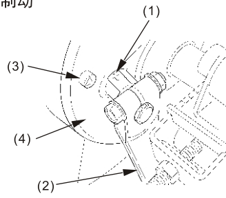
(1) 箭头 (2) 制动摇臂 (3) 指示符号 (4) 制动鼓盖
