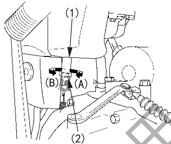
(1) 后制动灯开关 (2) 调节螺母
