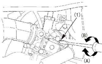
(1) 怠速调整螺钉 (A) 提高怠速 (B) 降低怠速
