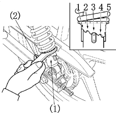
(1) 减震器
