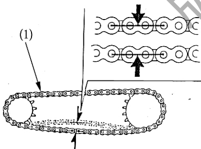
(1) 传动链
