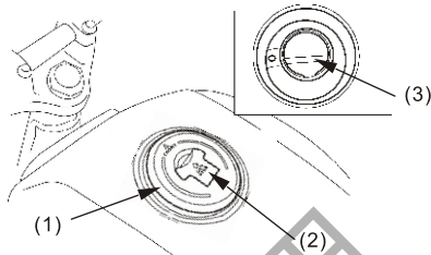
(1) 油箱盖 (2) 油箱盖盖板 (3) 油箱槽
