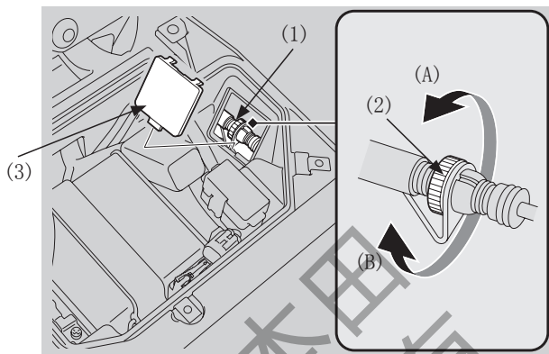
(1) 制动灯开关 (2) 调整螺母 (3) 调整盖
