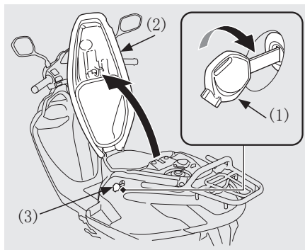
(1) 电源开关钥匙 (2) 鞍座 (3) 鞍座锁
