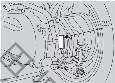
(2) 发动机编号
