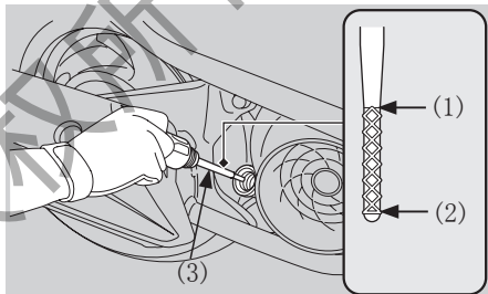
(1) 上限标记 (2) 下限标记 (3) 油标尺
