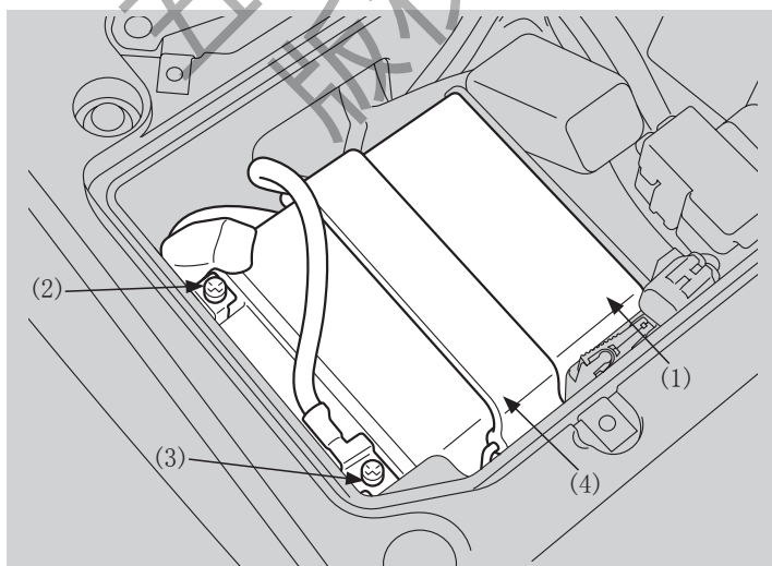
(1) 蓄电池 (2) 正极 (+) 端子 (3) 负极 (-) 端子 (4) 蓄电池箍带
