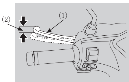
(1) 后制动手柄 (2) 后制动手柄自由行程
