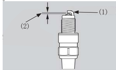
(1) 侧电极 (2) 火花塞间隙
