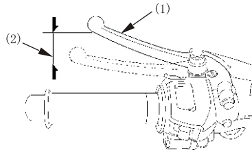
(1) 离合器手柄 (2) 离合器手柄自由行程
