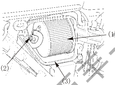
(1) 空气滤清器滤芯 (2) 螺钉 (3) 滤清器外壳
