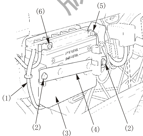
(1)通气管 (2)螺栓 (3)蓄电池 (4)电池托架 (5)正极端子 (6)负极端子
