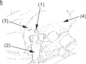
(1) 箭头 (2) 制动摇臂 (3) 指示符号 (4) 制动盘
