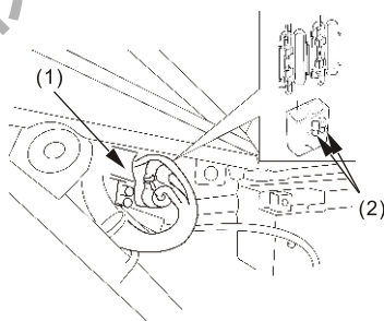
(1) 保险丝盒 (2) 备用保险丝
