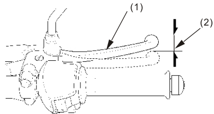
(1) 前制动手柄 (2) 前制动手柄自由行程
