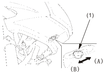
(1) 调整螺栓 (A) 调高 (B) 调低
