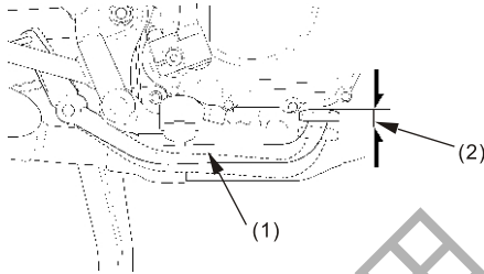
(1) 后制动踏板 (2) 后制动踏板自由行程
