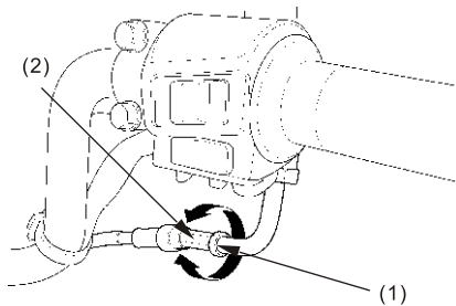
(1) 锁紧螺母 (2) 调整器
