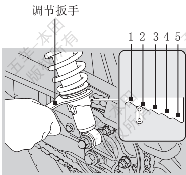
调节扳手
