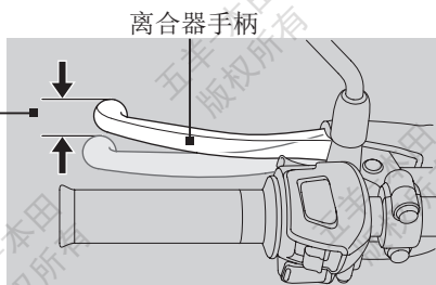
离合手柄自由行程
