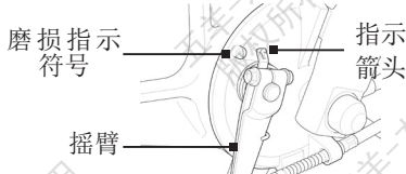
前制动鼓刹
