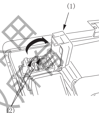
(1) 保险丝盒盖 (2) 备用保险丝
