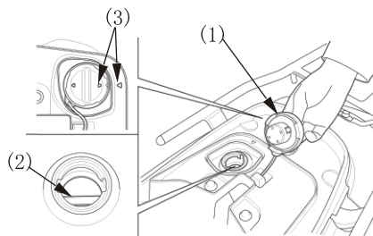
(1) 加油盖 (2) 油箱槽 (3) 箭头标记
