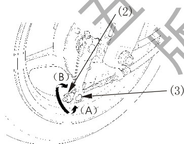
(2) 前制动调整螺母 (A) 增加 (3) 制动臂连接销 (B) 减少
