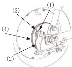
(1) 指示箭头 (2) 制动臂 (3) 参照标记 (4) 制动鼓盖
