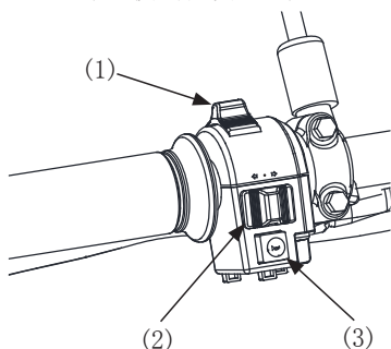
(1) 变光开关 (2) 左右转向开关 (3) 喇叭开关
