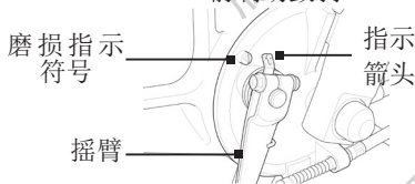
前制动鼓刹
