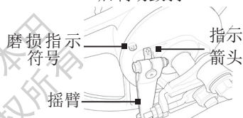
后制动鼓刹
