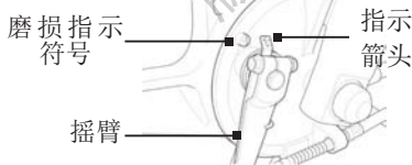
前制动鼓刹
